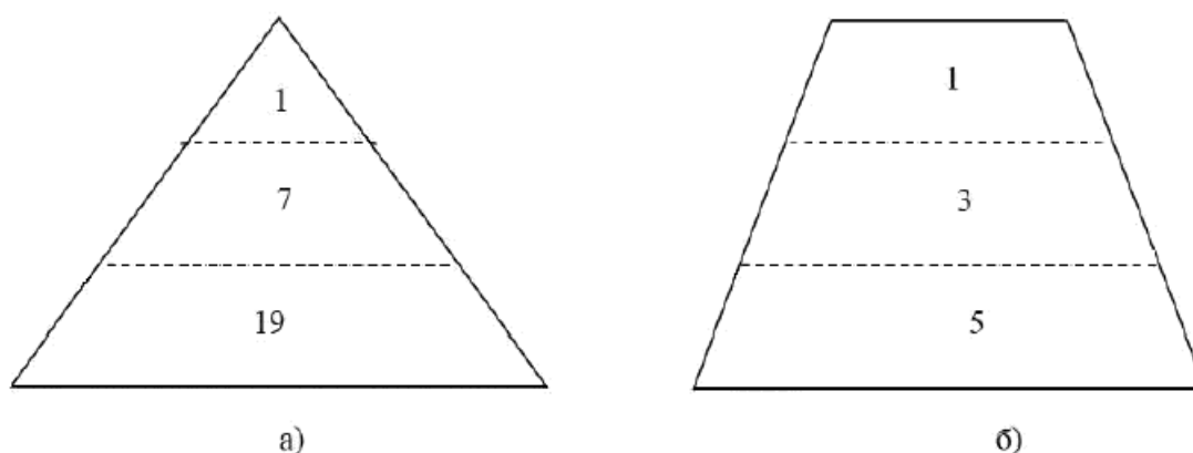
Рисунок 2 - Соотношения, в которых необходимо проводить отбор точечных проб из различных частей штабеля конусообразной а или призматической б форм
