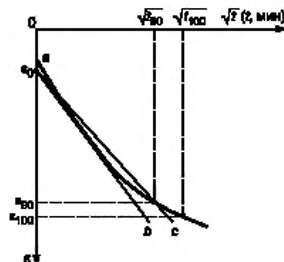
Рисунок Б.1 — График обработки кривой консолидации методом «корень квадратный из времени»
