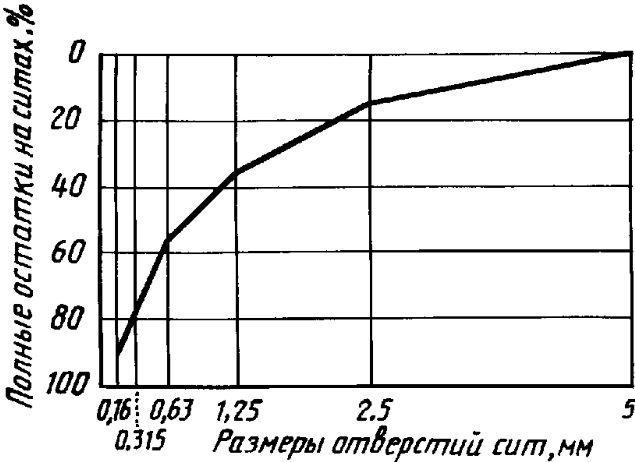
Кривая просеивания
