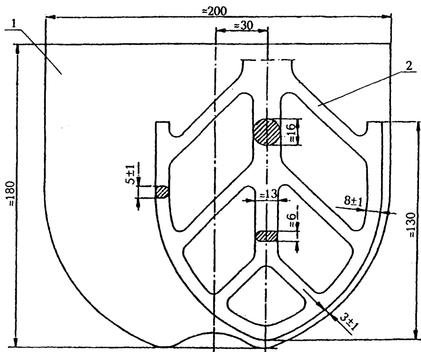
1 — чаша; 2 — лопасть
