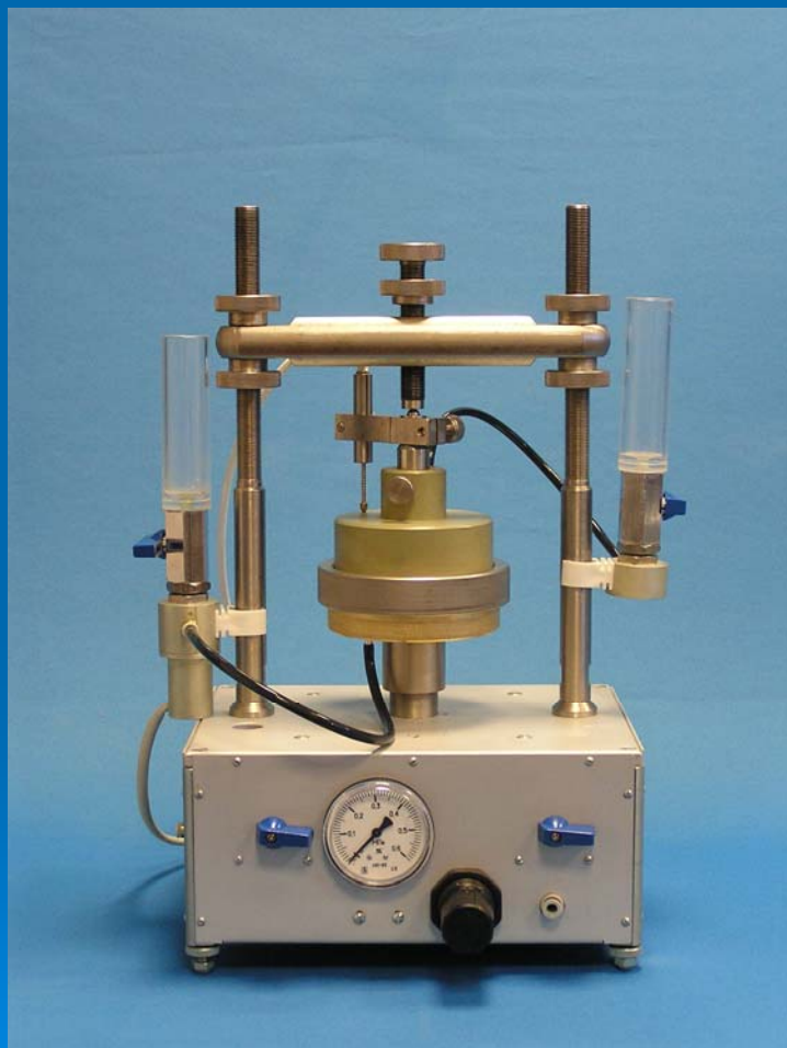
Компрессионный прибор
