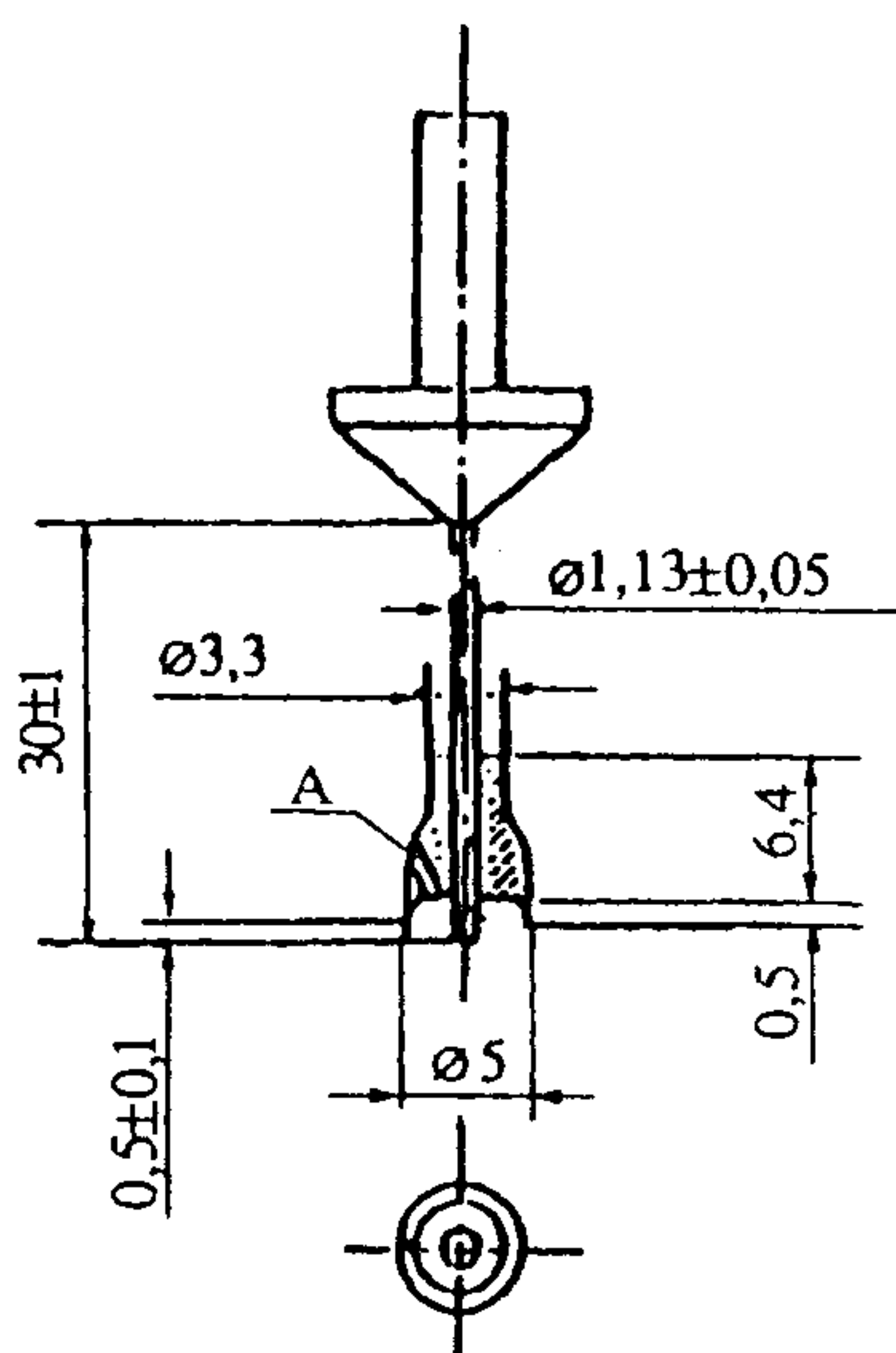
Рисунок 3 — Рабочая часть пестика
