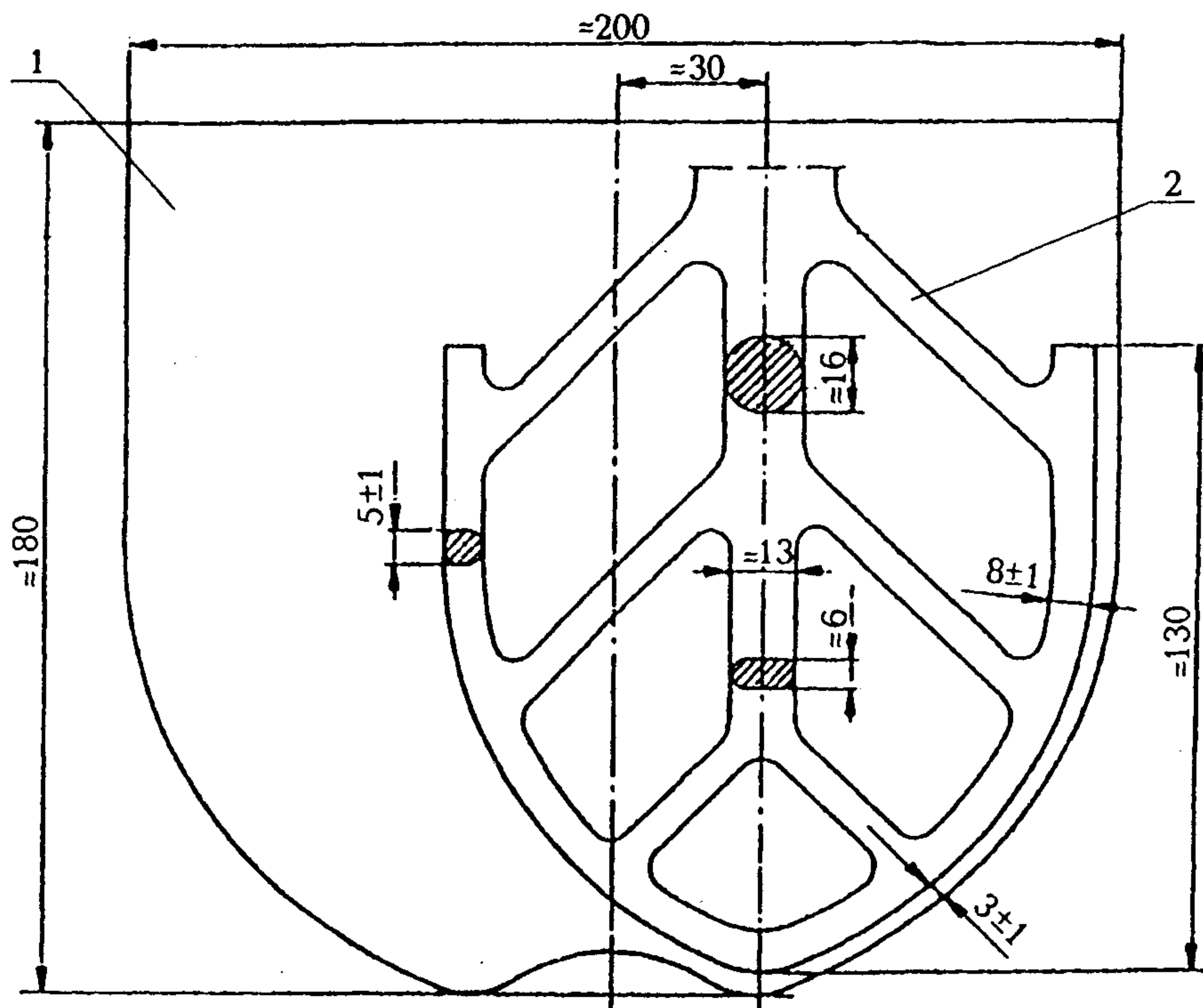
1 — чаша; 2 — лопасть
