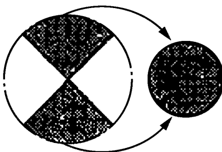
Рисунок А.1 — Сокращение пробы методом квартования
