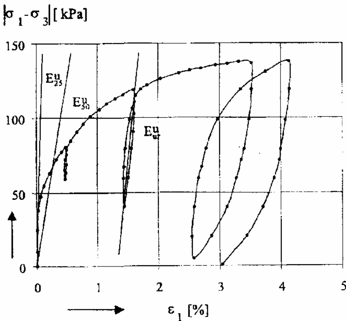
Рис. 16. Определение модуля деформации при разгрузке из результатов трехосных испытаний
