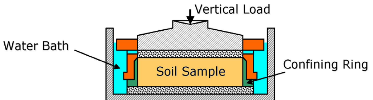
Рис. 17. Конструкция одометра
