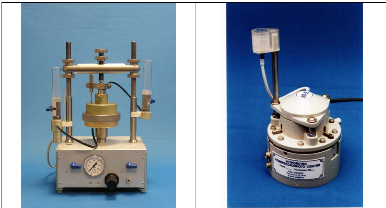
Рис. 18. Конструкция компрессионных приборов
