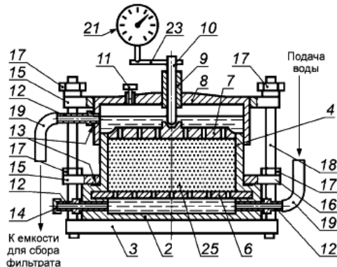
б) Для испытаний по схеме восходящего потока воды
