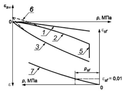
График 2 \varepsilon = f(p) (по схеме "трех кривых")
