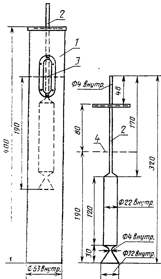
1 - цилиндр; 2 - пипетка; 3 - метка (1000 мл); 4 - уровень суспензии в цилиндре
