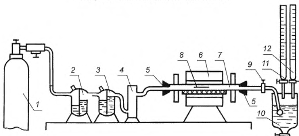
Схема установки для определения содержания серы
