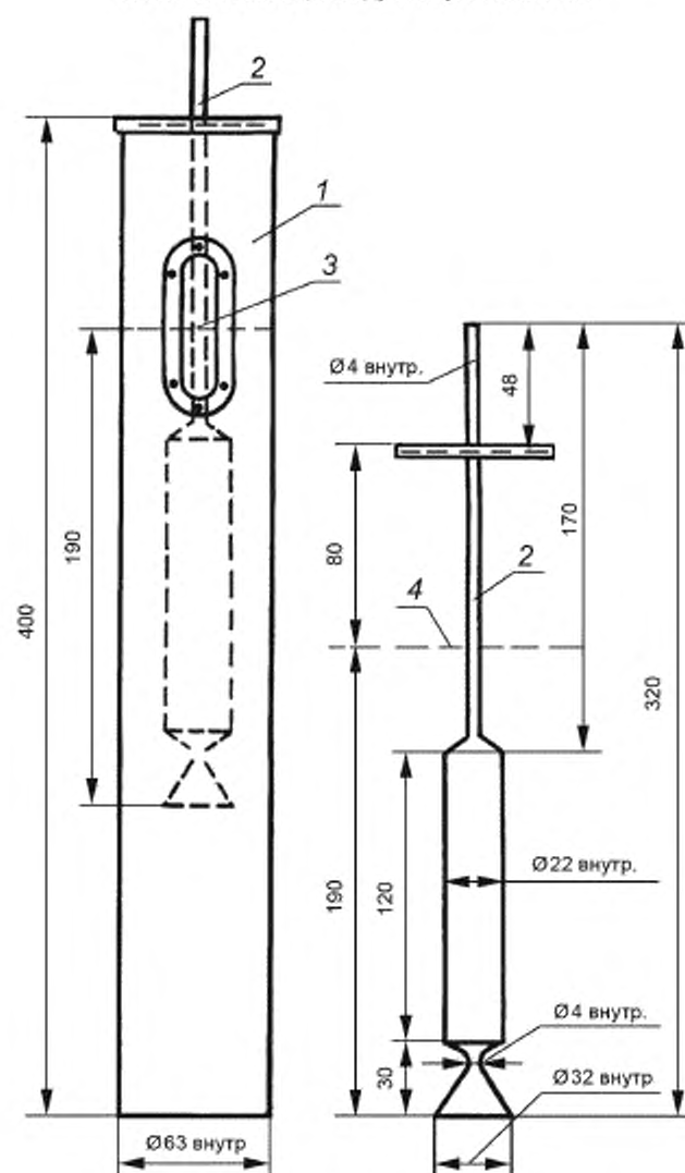
Металлический цилиндр и мерная пипетка
